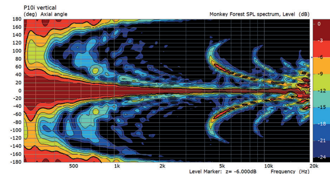
Vertikales Richtverhalten
